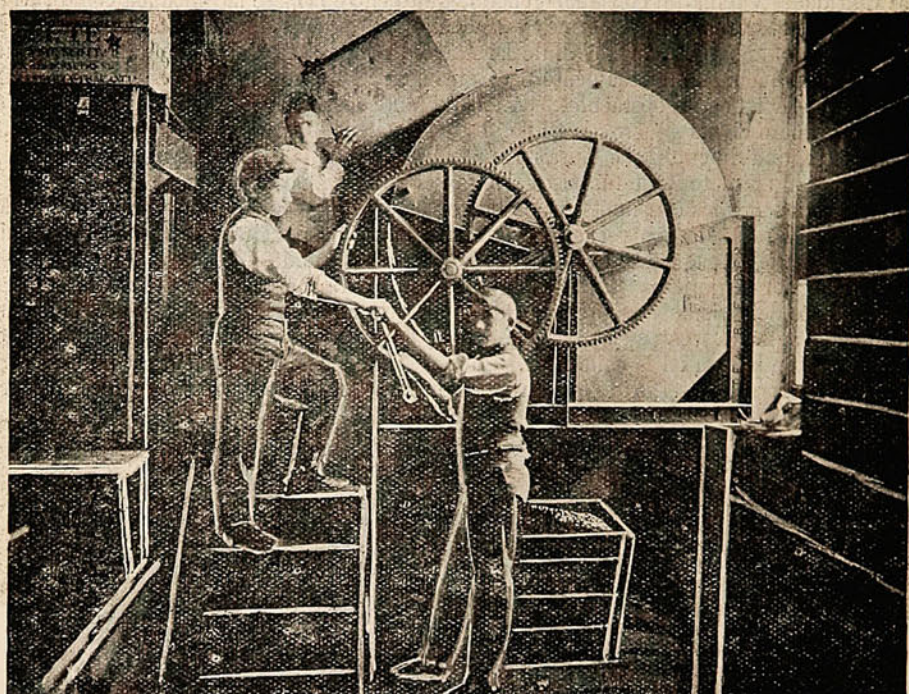
MÁQUINA PARA MEZCLAR TÉ.
